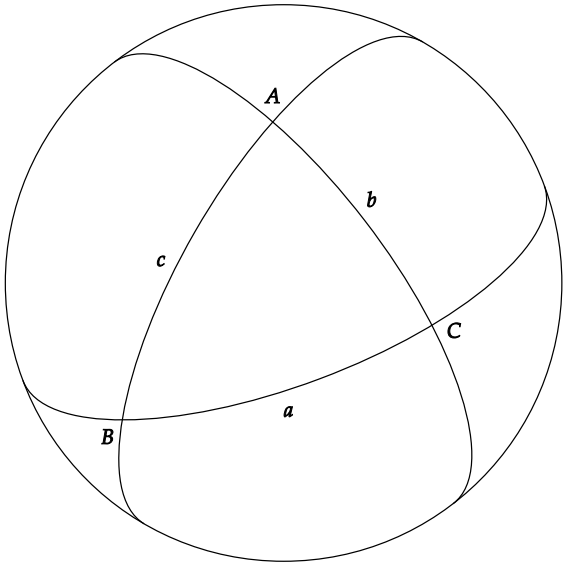
图 3.6: 球面三角形
